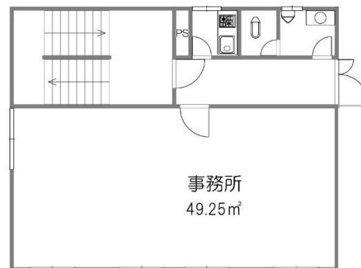
2階 平面図
