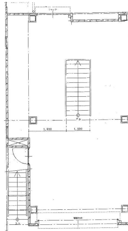
1階 平面図
